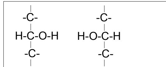
Fig. 5 Diferenciación en la posición de los -OH en los carbonos asimétricos de los monosacáridos.
