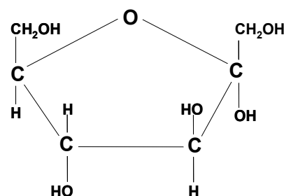
Fig. 12 Fórmula de la \alpha D fructofuranosa.
